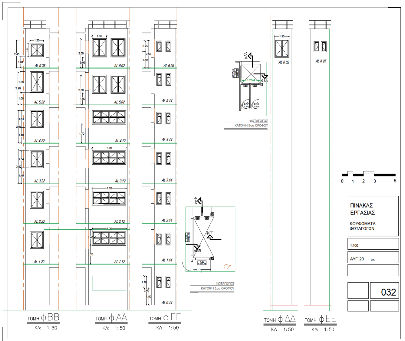
Πίνακας Εργασίας 3. Όψεις /Τομές Φωταγωγών
