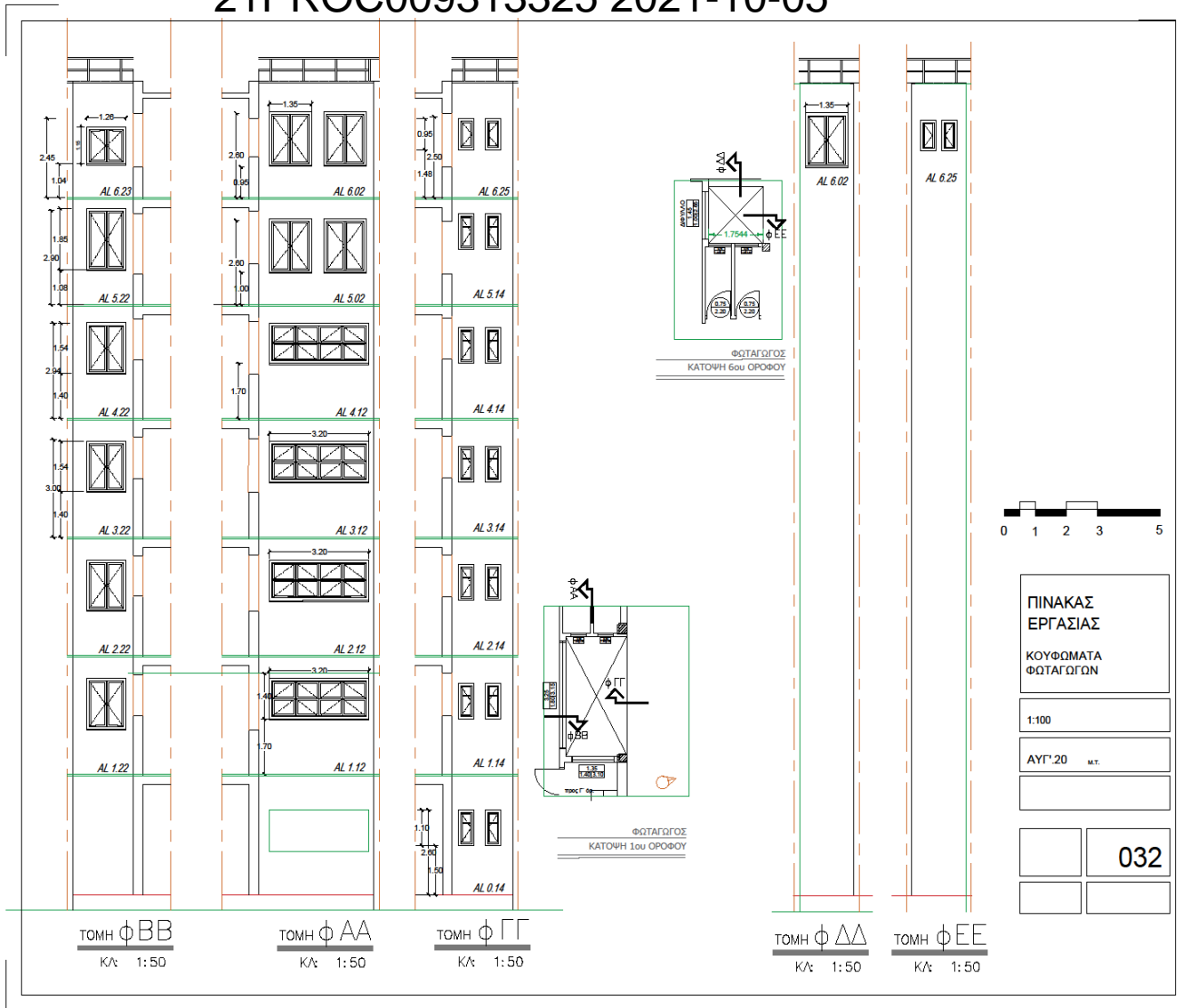
Πίνακας Εργασίας 3. Ώψεις /Τομές Φωταγωγών
